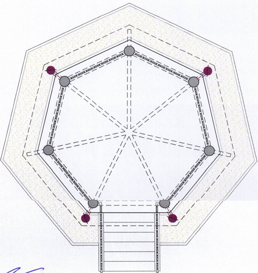
01 PLANTA DE PONTOS ELÉTRICOS-CORETO escala: 1/50
