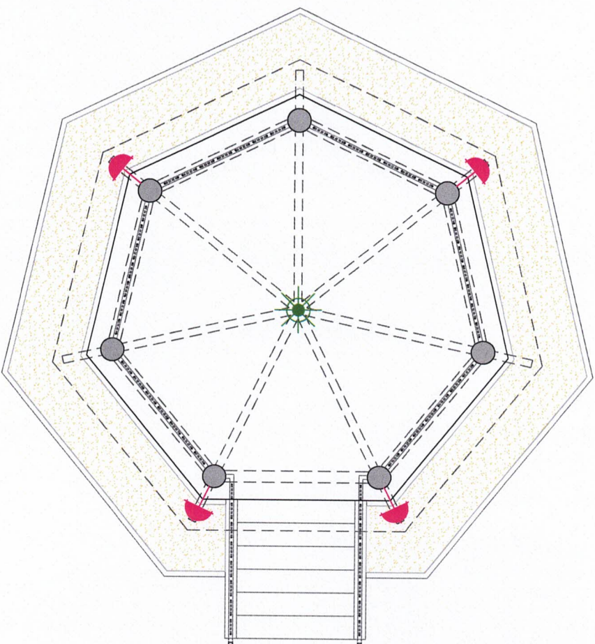
02 PLANTA DE PONTOS LUMINOTÉCNICOS-CORETO escala: 1/50
