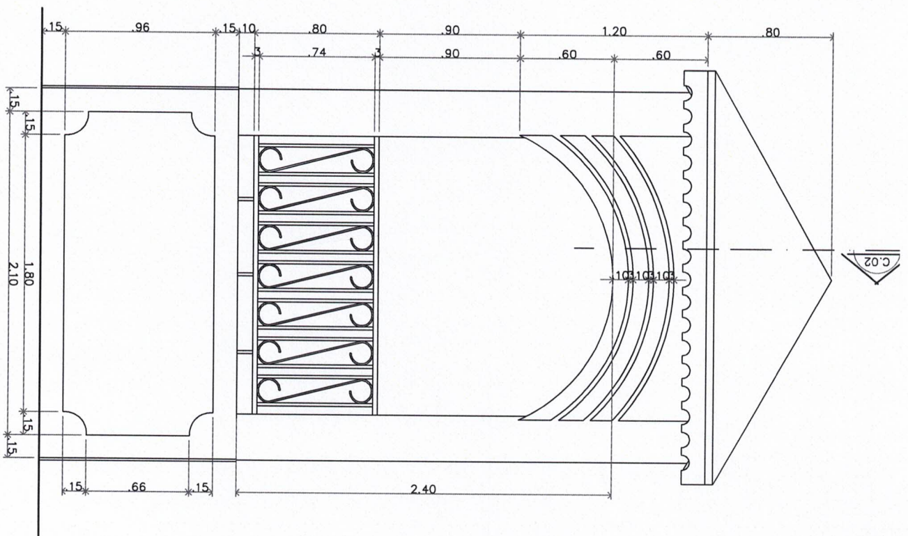
01 DETALHES CONSTRUTIVOS - VISTA 02 escala: 1/25
