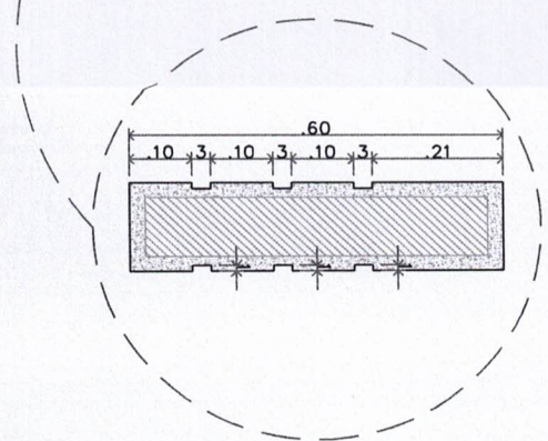
DETALHE ALVENARIA EM ARCO ESC: 1/10
